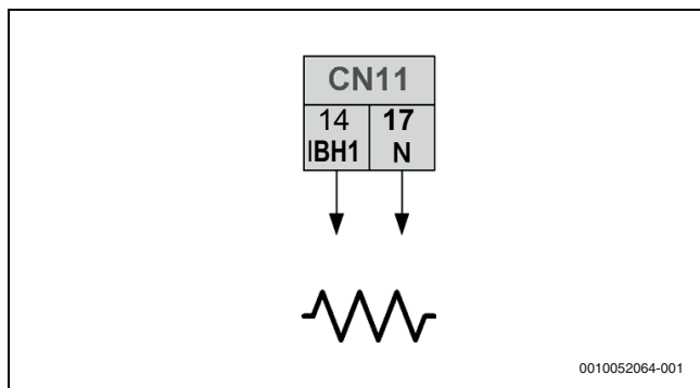
Afb. 88 Externe back-upverwarming
