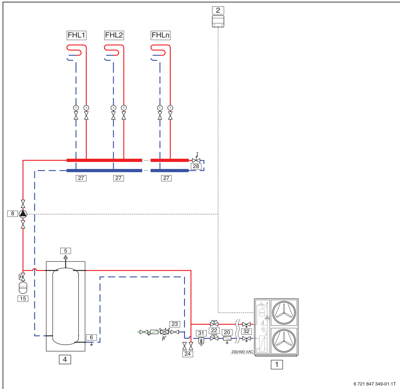
Afb. 19 Buitenunit met één of meerdere cv-groepen (CS2000AWF 18-30 R-T)
