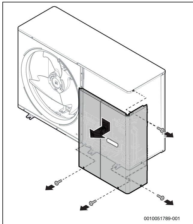
Afb. 48 Verwijder de beveiligingen
