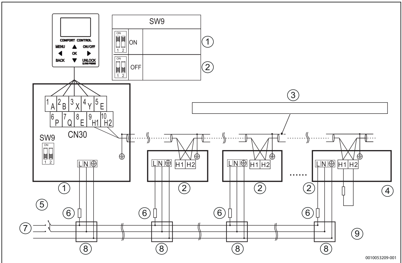
Afb. 104 Aansluitschema van het elektrische regelsysteem voor het cascadesysteem (1N ~)
