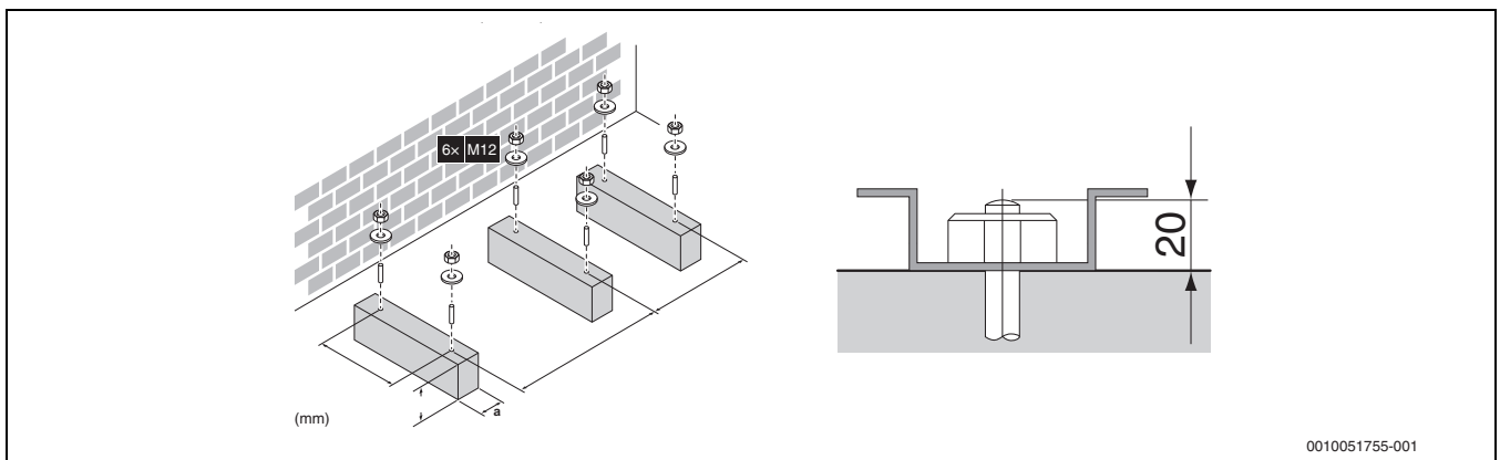
Afb. 41 Montage op de grond
