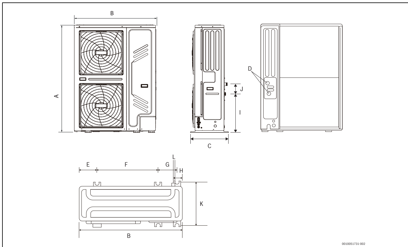
Afb. 34 Afmetingen CS2000AWF 18 R-T tot CS2000AWF 30 R-T
