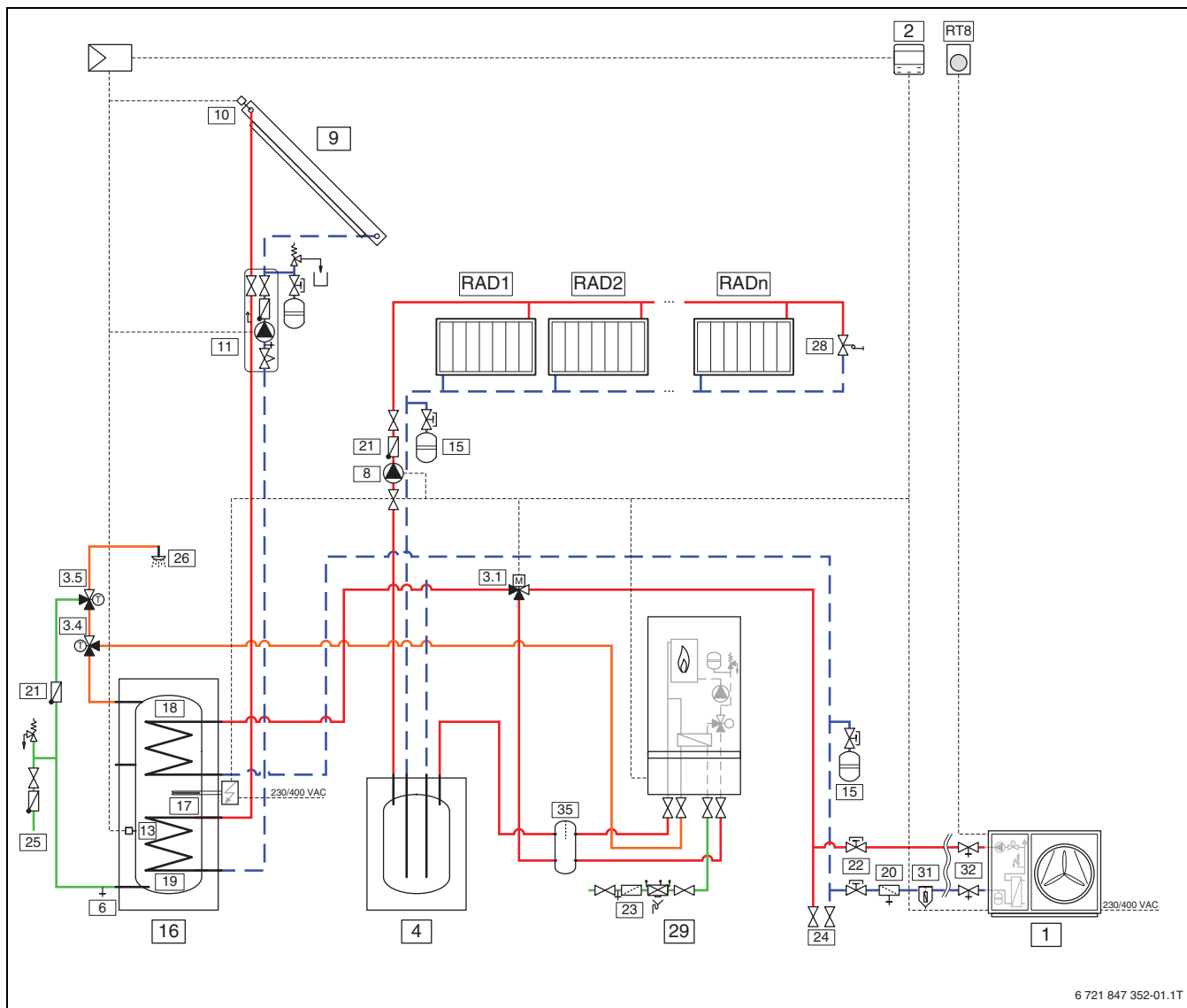
Afb. 22 Buitenunit met één of meerdere cv-groepen, externe bijverwarming, boiler en zonnestelsysteem (CS2000AWF 4-6 R-S, CS2000AWF 8-10 R-S, CS2000AWF 12-16 R-S/T)
