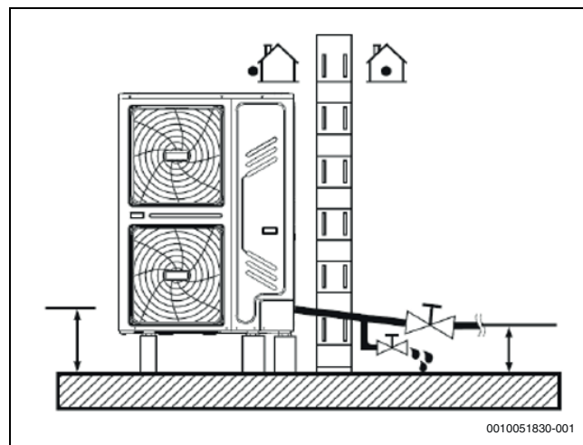
Afb. 54 Vorstbeveiliging watercircuit
