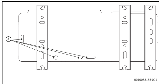
Afb. 47 Afvoeropeningen
