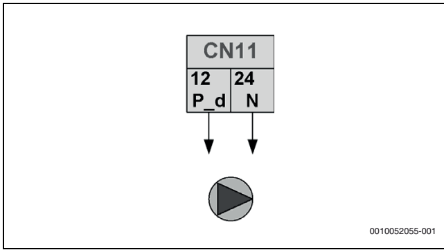
Afb. 80 Warmwaterpomp, type 2 regelsignaal
