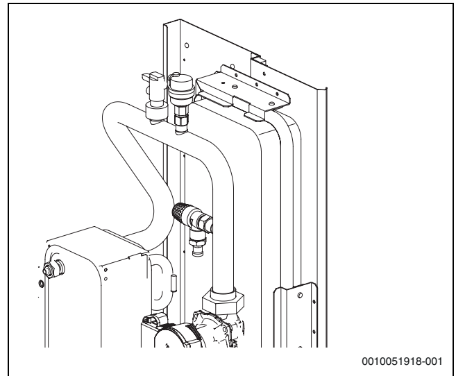
Afb. 60 Vullen / bijvullen met water
