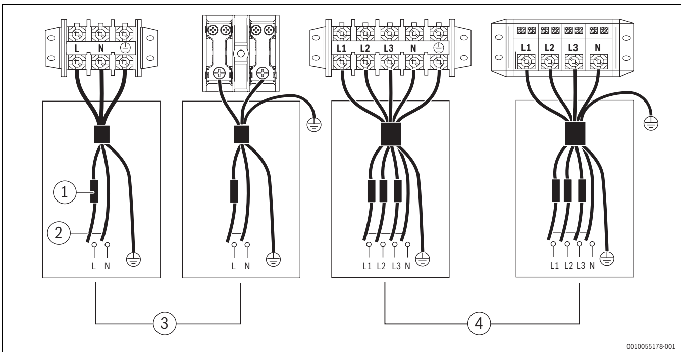
Afb. 72 Compressorcompartiment en elektrische onderdelen: XT1
