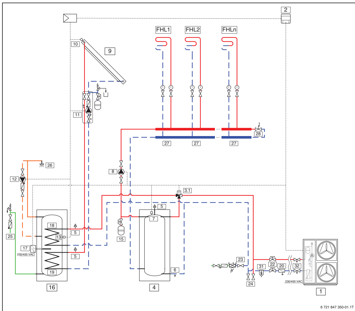
Afb. 20 Buitenunit met één of meerdere cv-groepen, boiler en zonnestelsysteem (CS2000AWF 18-30 R-T)
