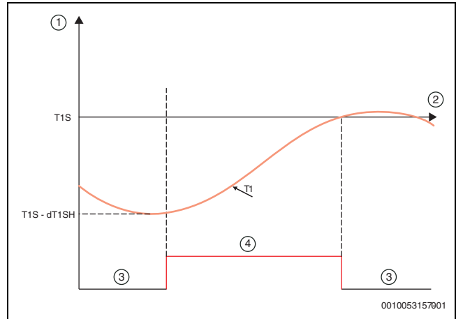
Afb. 125 Verwarmingsbedrijf - wateraanvoertemperatuur ( T1 )
