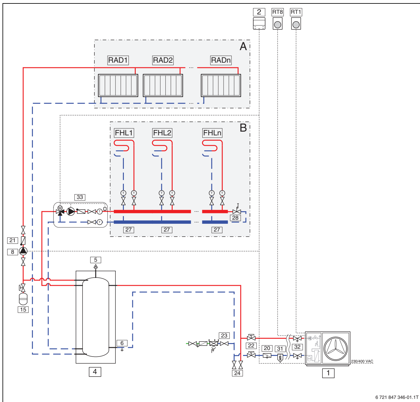
Afb. 18 Buitenunit met één of meerdere cv-groepen, vloerverwarming en radiatoren (CS2000AWF 4-6 R-S, CS2000AWF 8-10 R-S, CS2000AWF 12-16 R-S/T)
