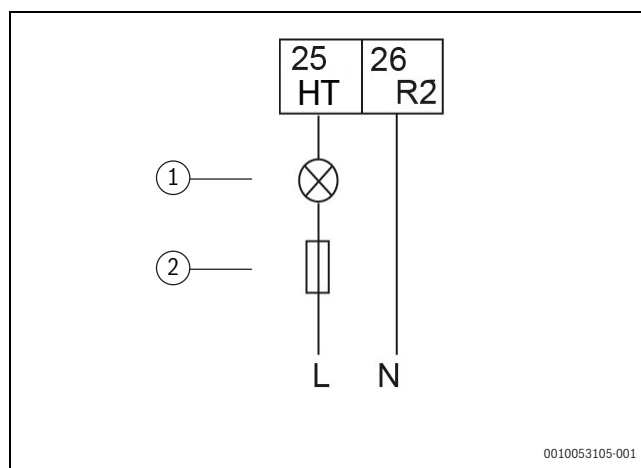
Afb. 74 TYPE 1 stuursignaal
