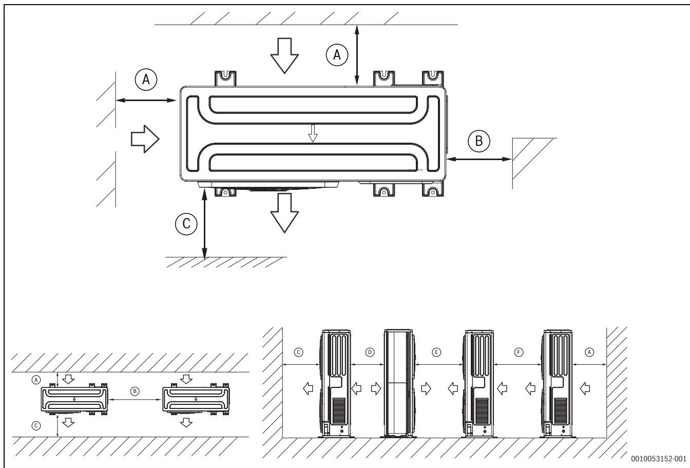
Afb. 36 Minimale afstanden
