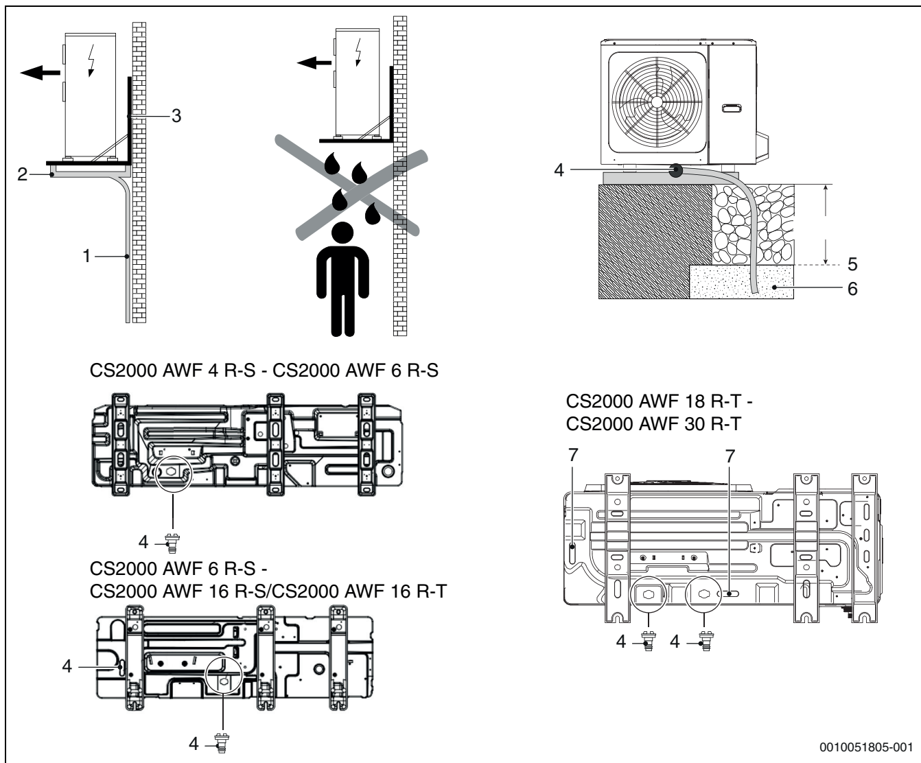
Afb. 49 Condensafvoer
