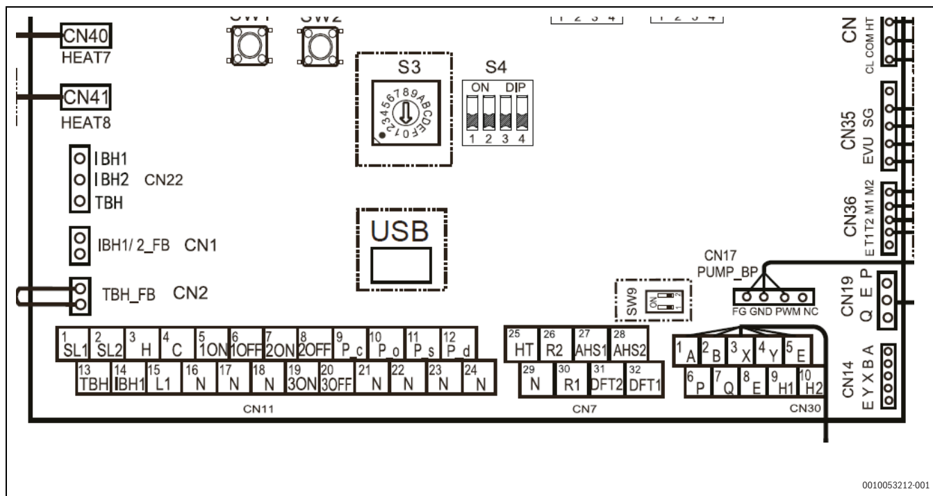
Afb. 73 Klemmenblok aansluiten
