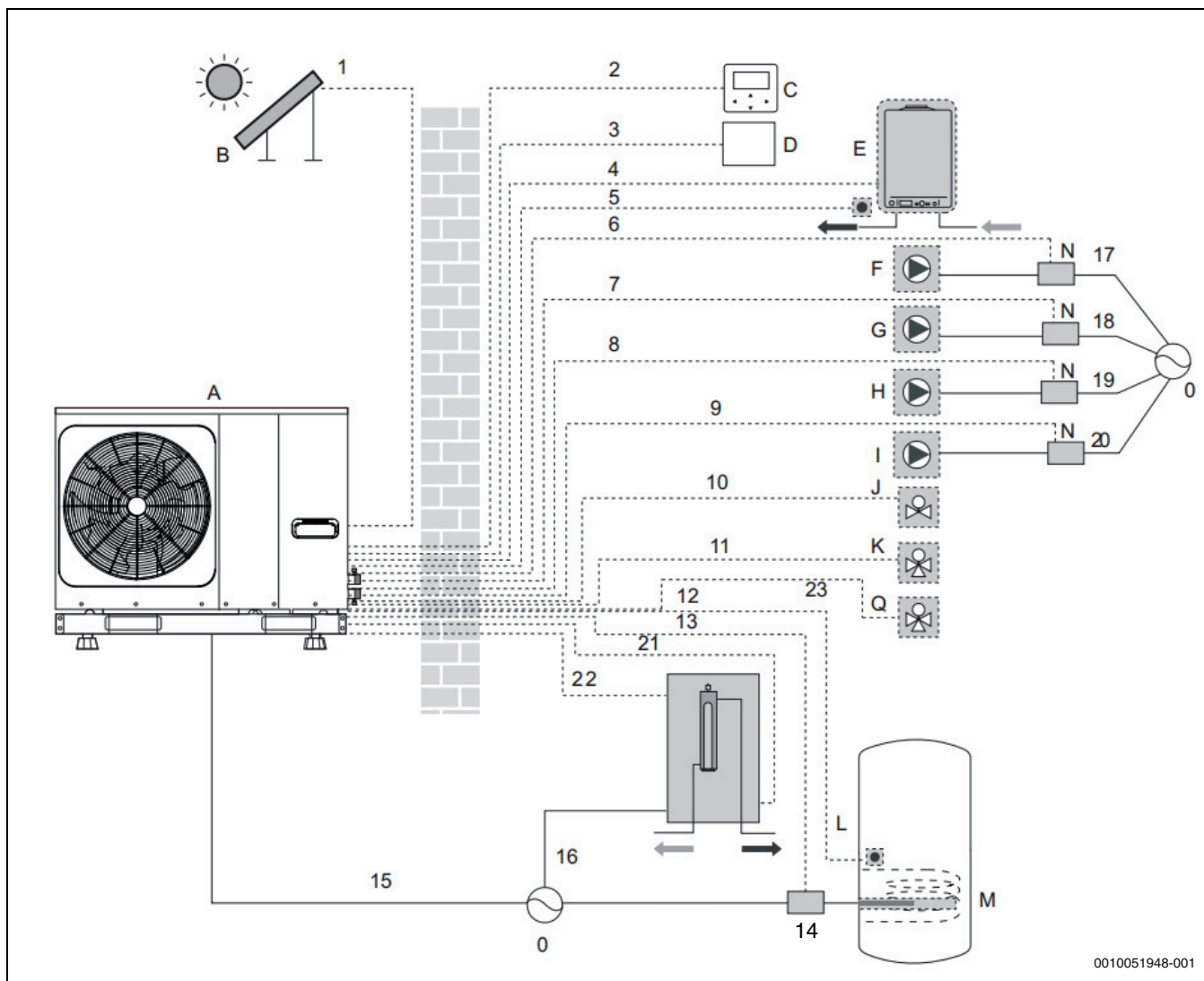
Afb. 61 Algemeen schema
