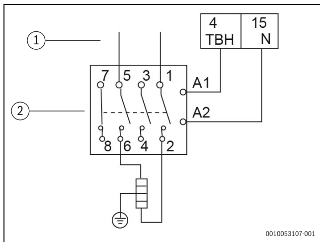
Afb. 75 TYPE 2 stuursignaal
