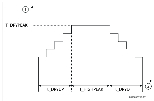
Afb. 143 Diagram droogcyclus
