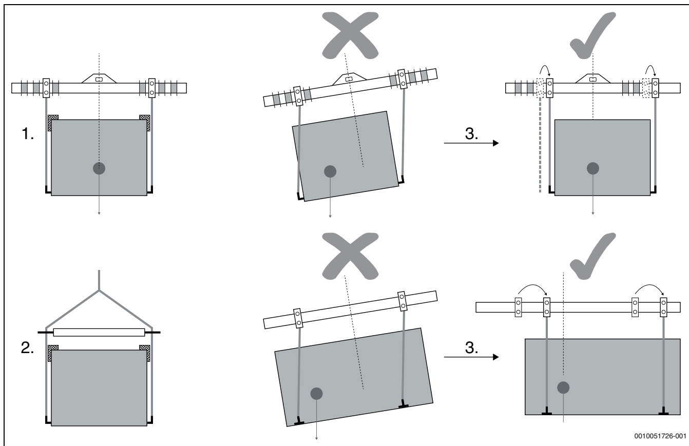
Afb. 29 Hijsen
