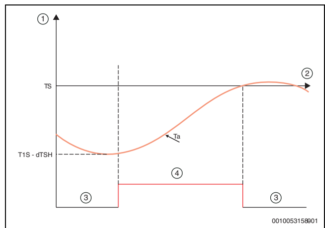
Afb. 126 Verwarmingsbedrijf - luchttemperatuur ( Ta )
