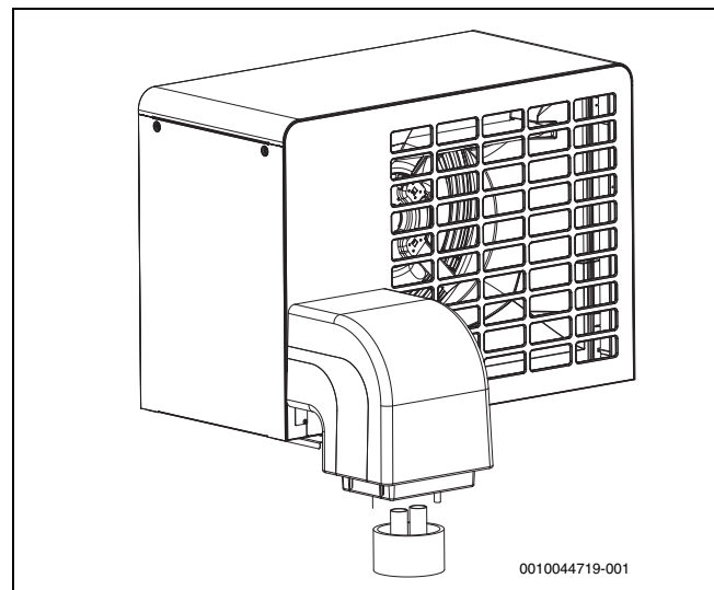
Afb. 21 Installatieset, vloermontage
