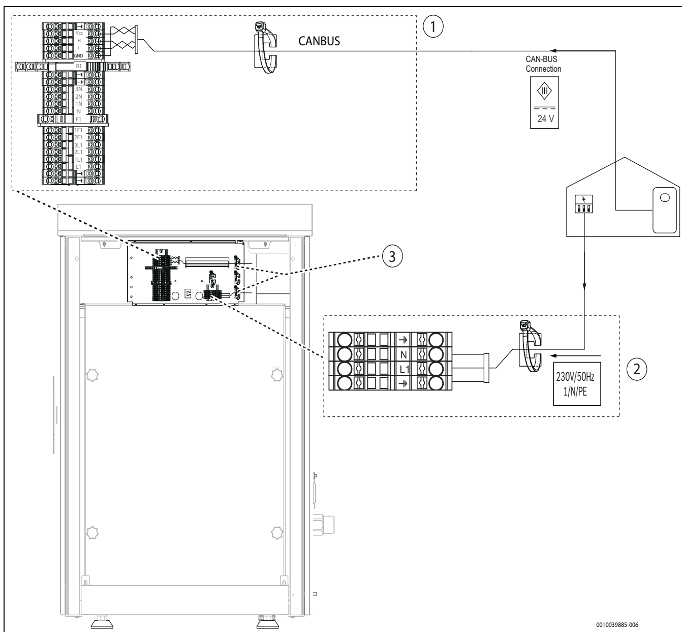
Afb. 37 Aansluitkast
