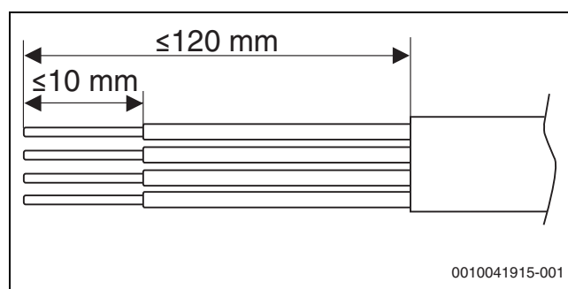
Afb. 35 Ader strippen CAN-BUS
