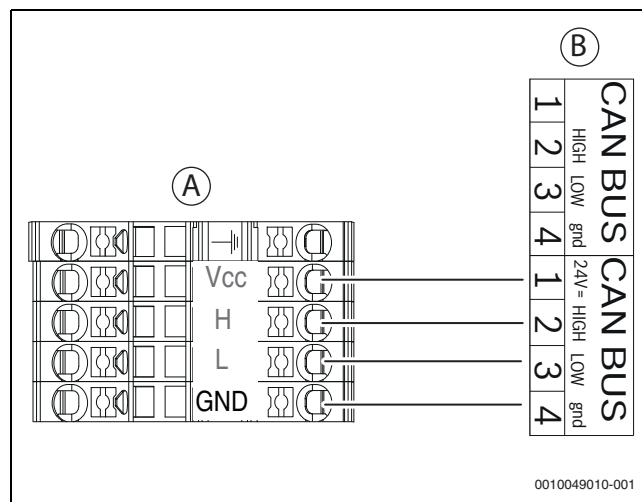
Afb. 34 CAN-BUS warmtepomp - binnenunit
