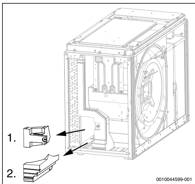
Afb. 41 EPP-onderdelen
