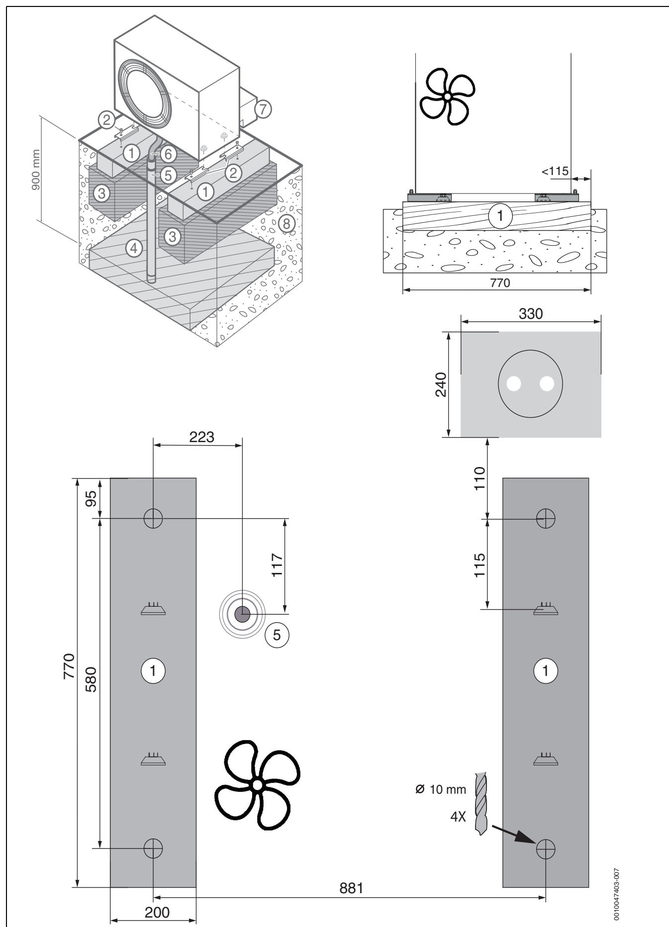
Afb. 28 Funderingsschema, alternatief 1
