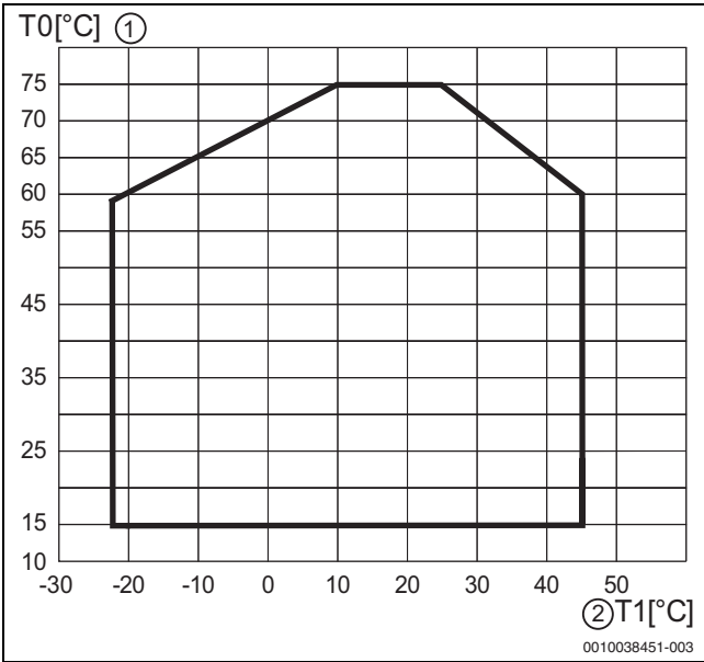
Afb. 44 Warmtepomp in verwarmingsmodus zonder boosterverwarming
