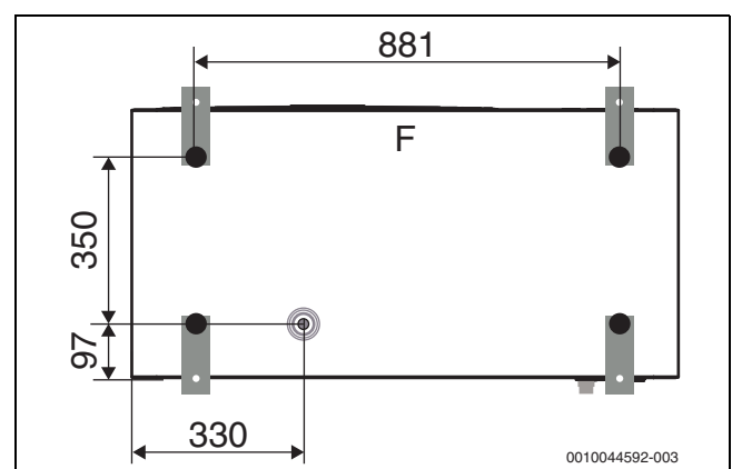
Afb. 6 Afstanden tot aftapaansluiting, aanzicht onderkant
