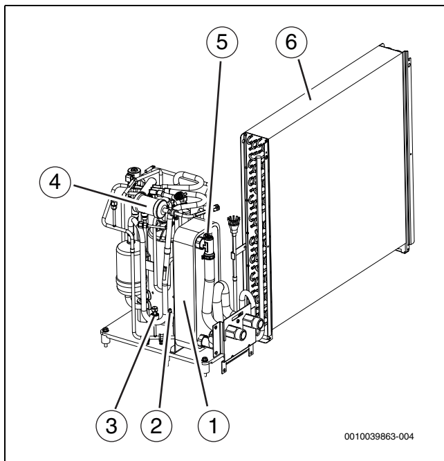
Afb. 3 Productoverzicht achteraanzicht
