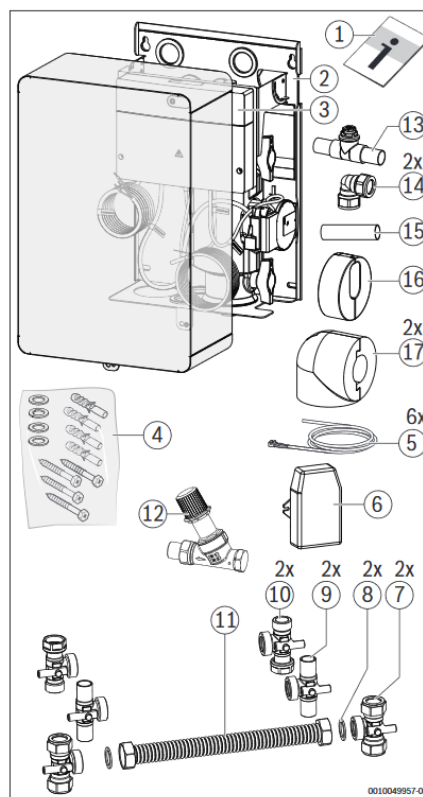
Afb. 1 Leveringsomvang CSH5800iAW O
