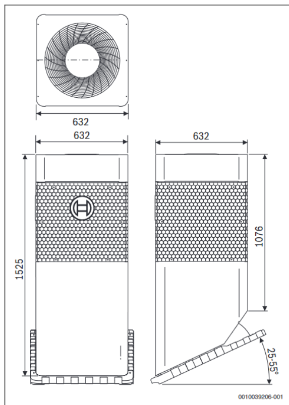
Afb. 4 Afmetingen en aansluitingen warmtepomp.
