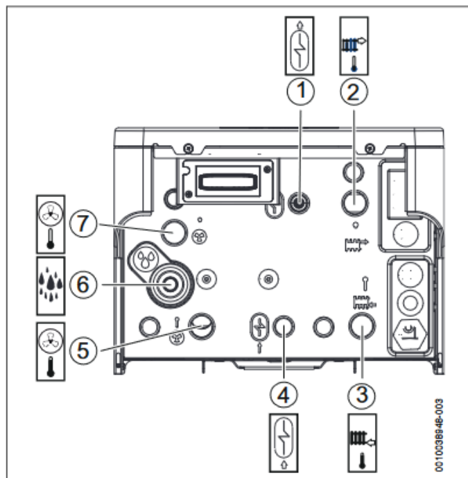
Afb. 6 Aansluiting leidingwerk
