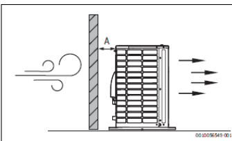
Afb. 19 Vrijstaande warmtepomp
