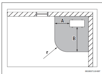
Afb. 10 Veiligheidszone op de grond geplaatst in een hoek, bovenaanzicht
