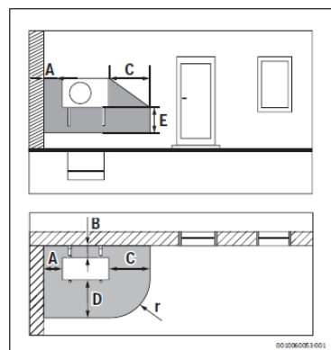
Afb. 13 Veiligheidszone, wandmontage warmtepomp
