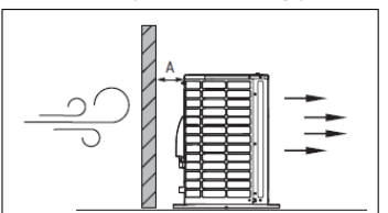
Afb. 19 Vrijstaande warmtepomp
