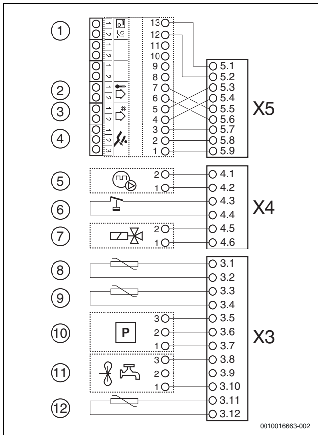
Afb. 37 24 V-deel
