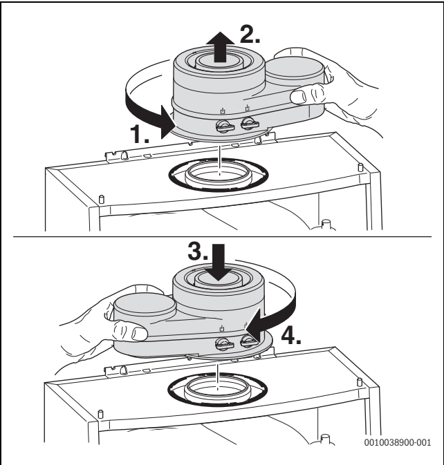
Afb. 6 Omdraaien rookgasafvoeradapter
