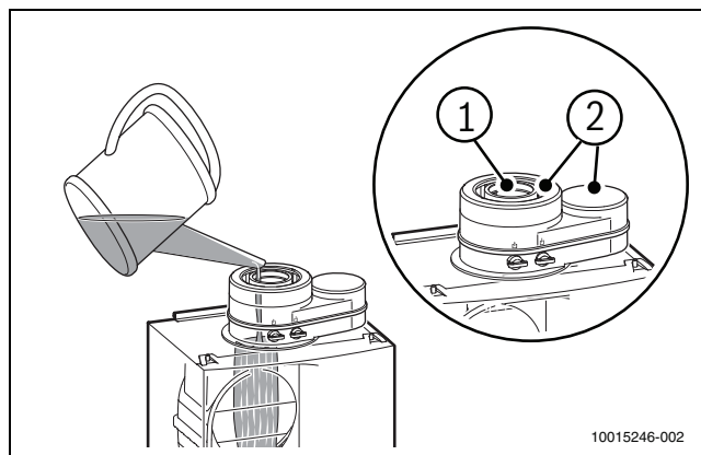
Afb. 22 Vullen toestelsifon
