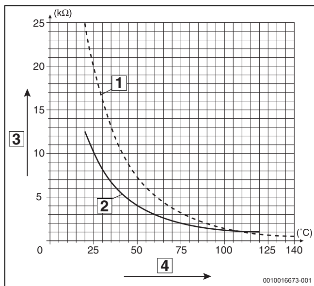
Afb. 40 Weerstandsgrafiek NTC-sensoren
