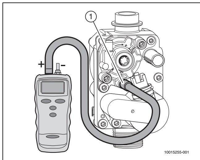
Afb. 32 Meten dynamische gasvoordruk
