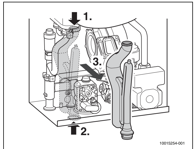
Afb. 31 Verwijderen toestelsifon
