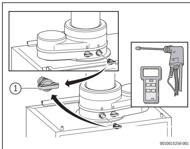
Afb. 33 Verwijderen afdekdop
