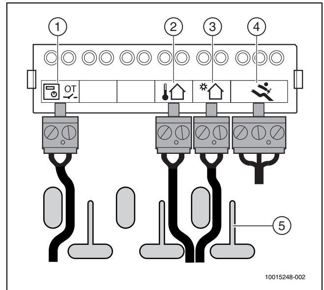
Afb. 25 Aansluiten componenten
