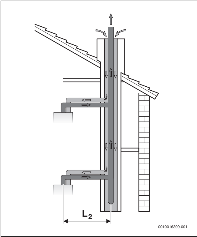
Afb. 18 Collectieve rookgasafvoer met parallelle leiding: C 43
