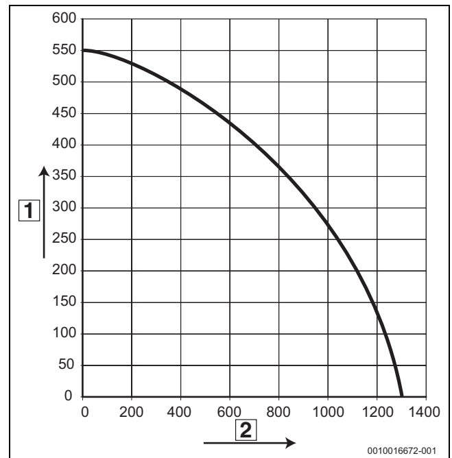
Afb. 39 Restopvoerhoogte
