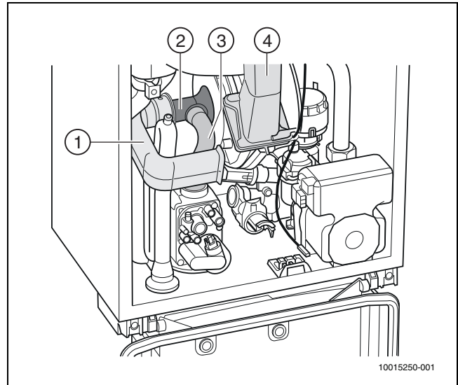
Afb. 27 Demonteren gas-luchtunit
