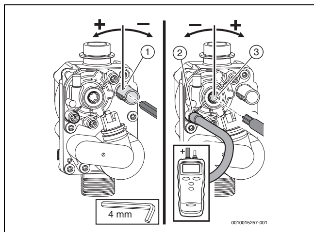
Afb. 35 Afstellen gasregelblok
