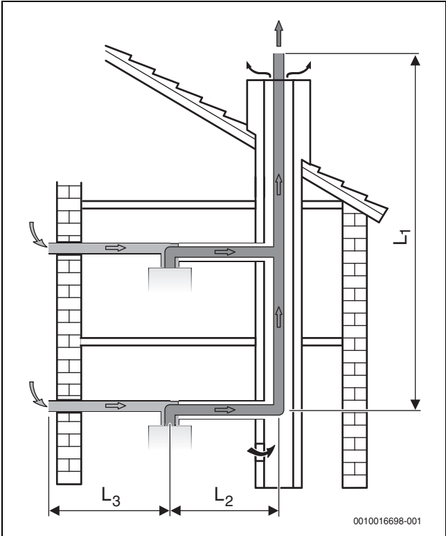
Afb. 19 Collectieve rookgasafvoer met parallelle leiding: C 83
