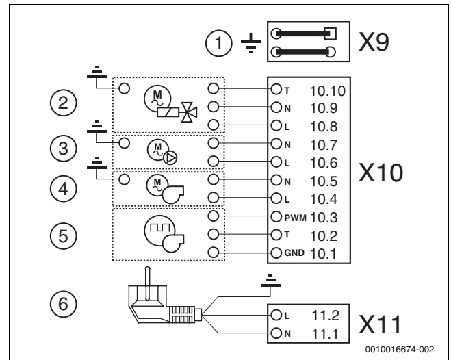
Afb. 38 230 V-deel
