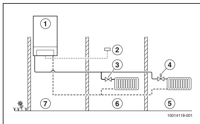
Afb. 23 Regelprincipe ruimteregeling
