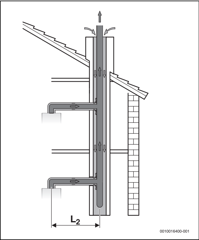
Afb. 17 Collectieve rookgasafvoer met concentrische leiding: C 43 , C (10)3 , C (11)3
